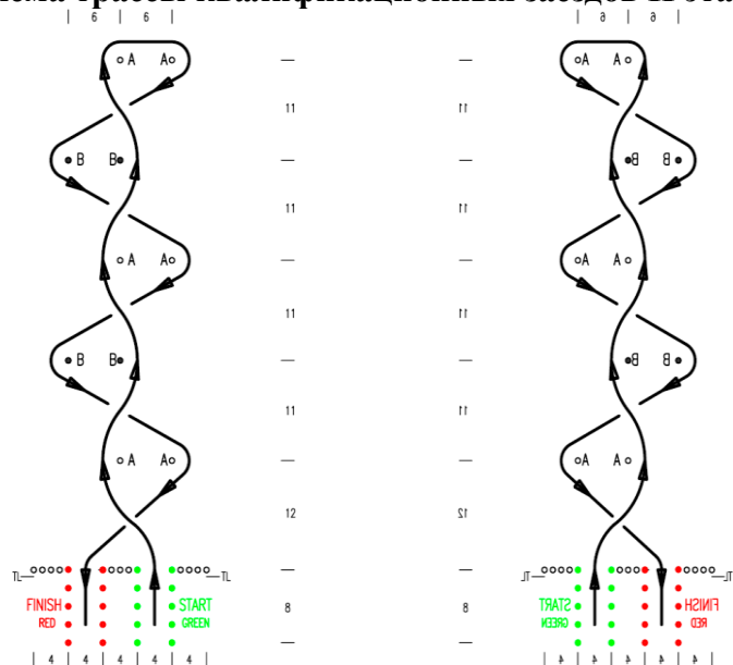
Схема трассы квалификационных заездов II этапа:
